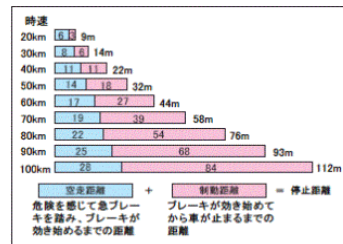
図3 スピードと停止距離の目安
